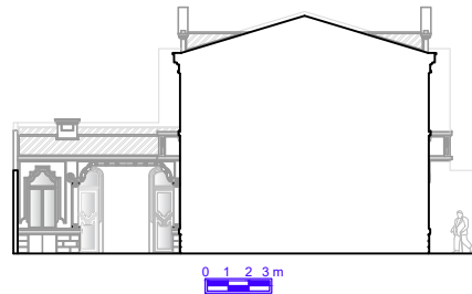
Elevation 02
