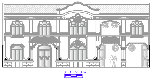
Elevation 01
